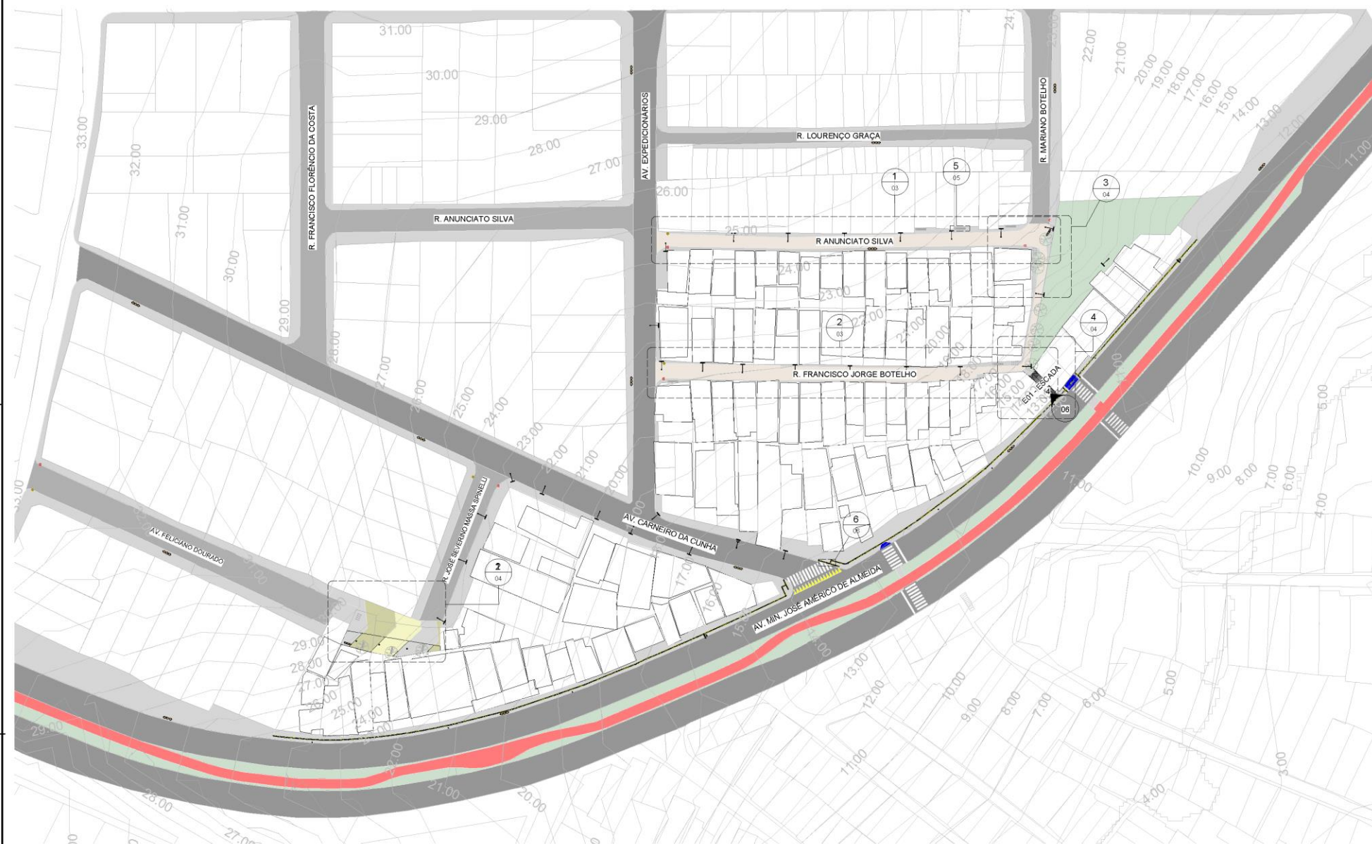
1 PLANTA DE SITUAÇÃO PROPOSTA
